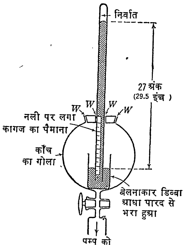
चित्र 8—बैरोमीटर के संचय से ऊपर उपस्थित हवा को हटाने वाले बॉयल के उपकरण का चित्र। काँच का गोला पम्प का ऊपरी भाग है। W उन स्थानों को बताता है, जिस जगह सीलिंग वैक्स लगाया गया। जब पम्प को चलाया जाता है तो पारद के स्तम्भ की ऊँचाई कम हो जाती है।
